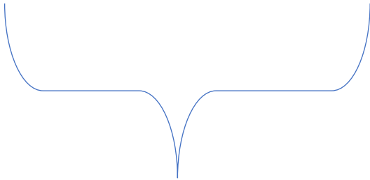
Les 4 planètes telluriques
