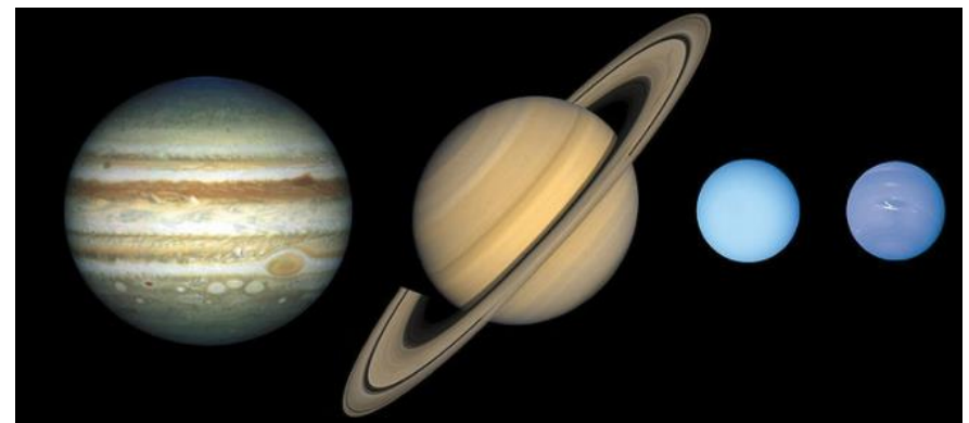
Les 4 planètes géantes
